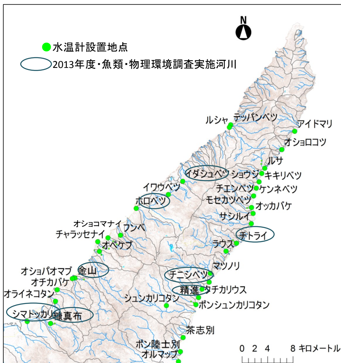
図 4. 水温計の設置と魚類・物理環境調査を行った位置図
