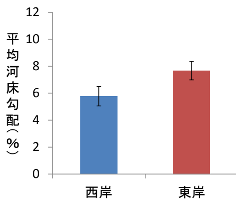
図 18. 西岸と東岸の河川勾配
