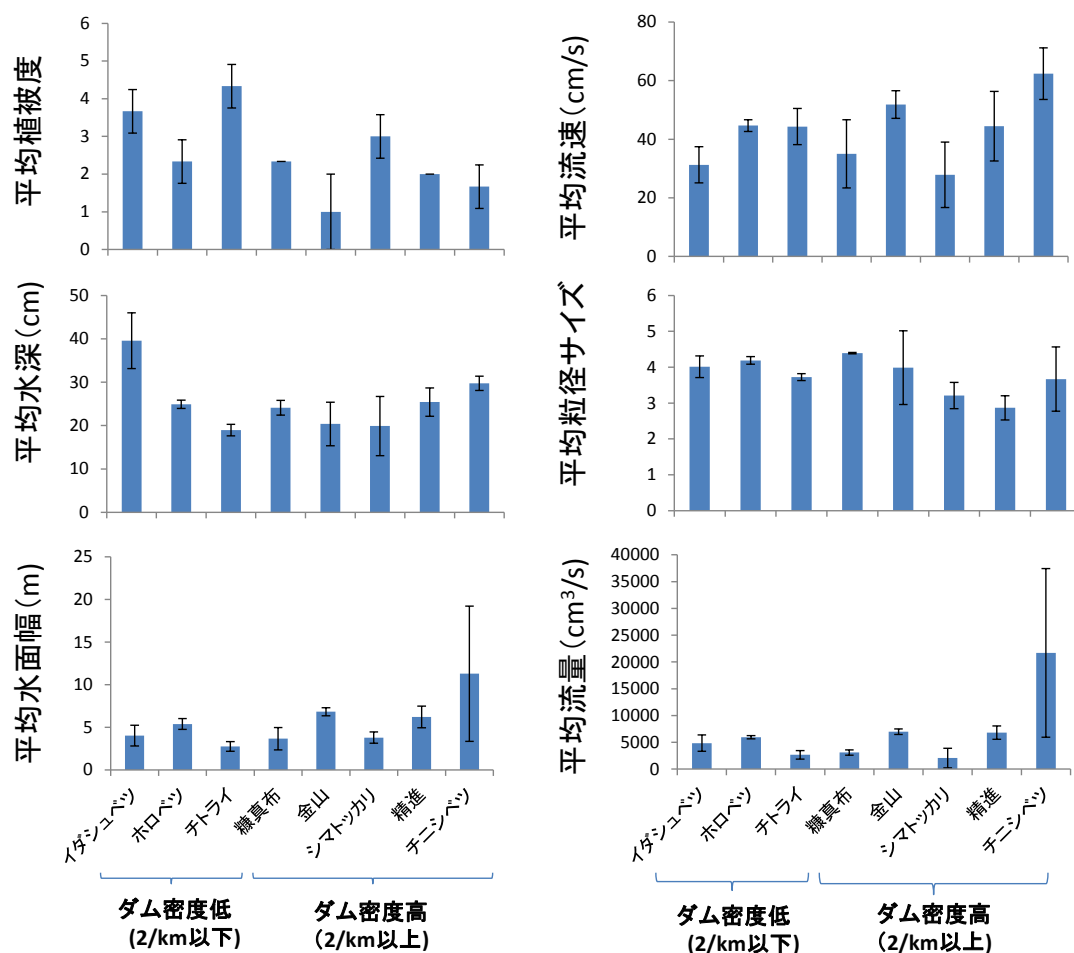
図 28. H25（2013）年に物理環境調査を行った 8 河川の物理環境 6 項目のデータ
