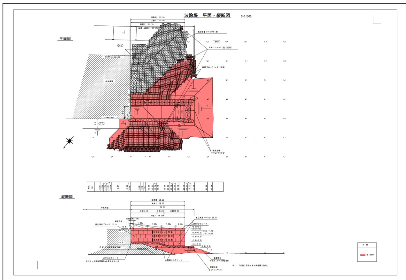
構造物（または、平面図） 波除堤
