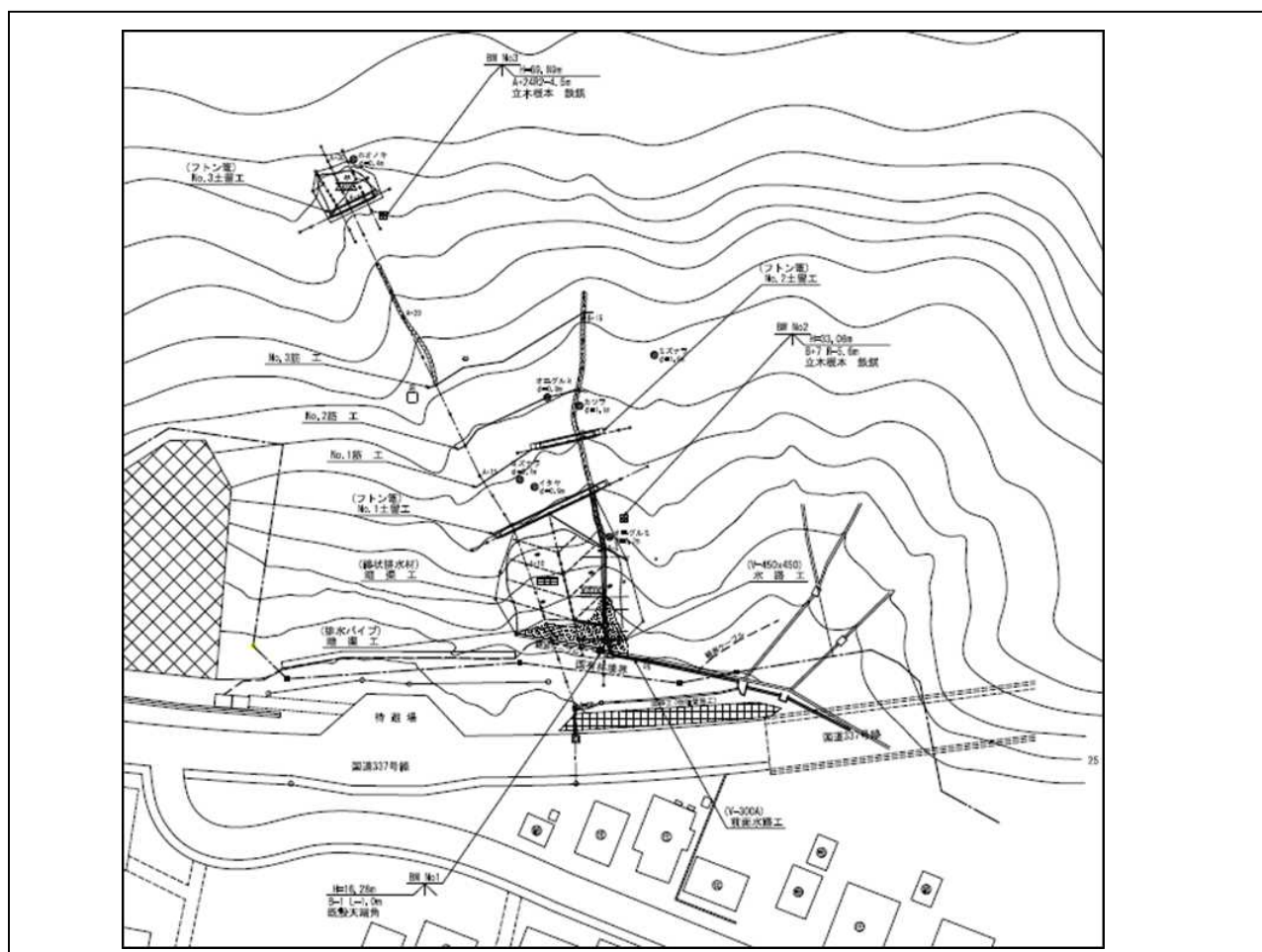
平面図
