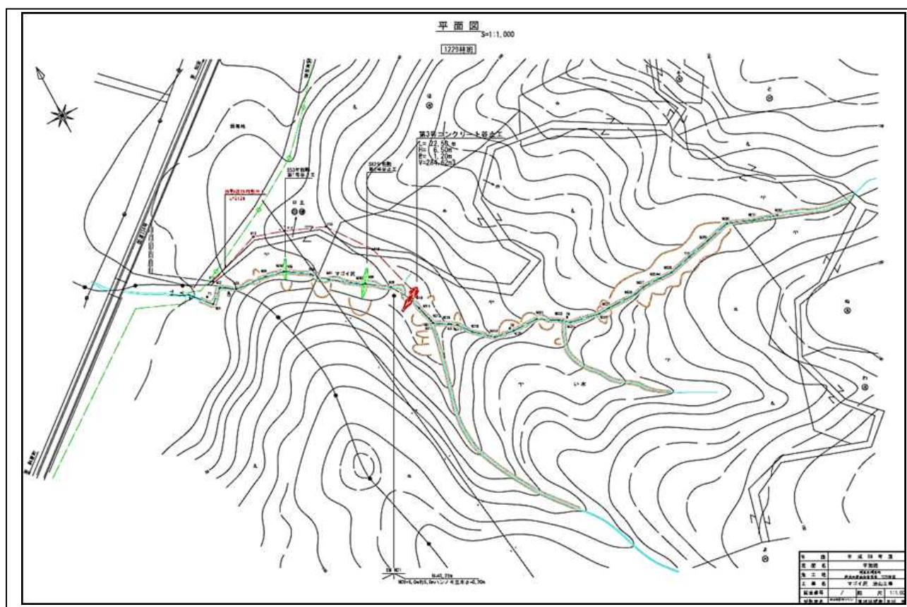
平面図
