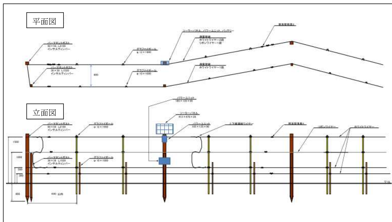
平面図及び立面図
