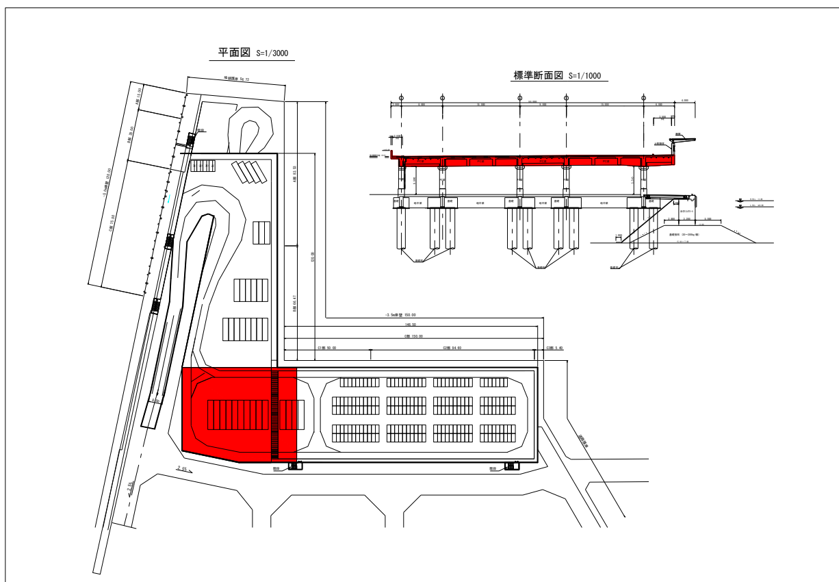
構造図（または、平面図）
