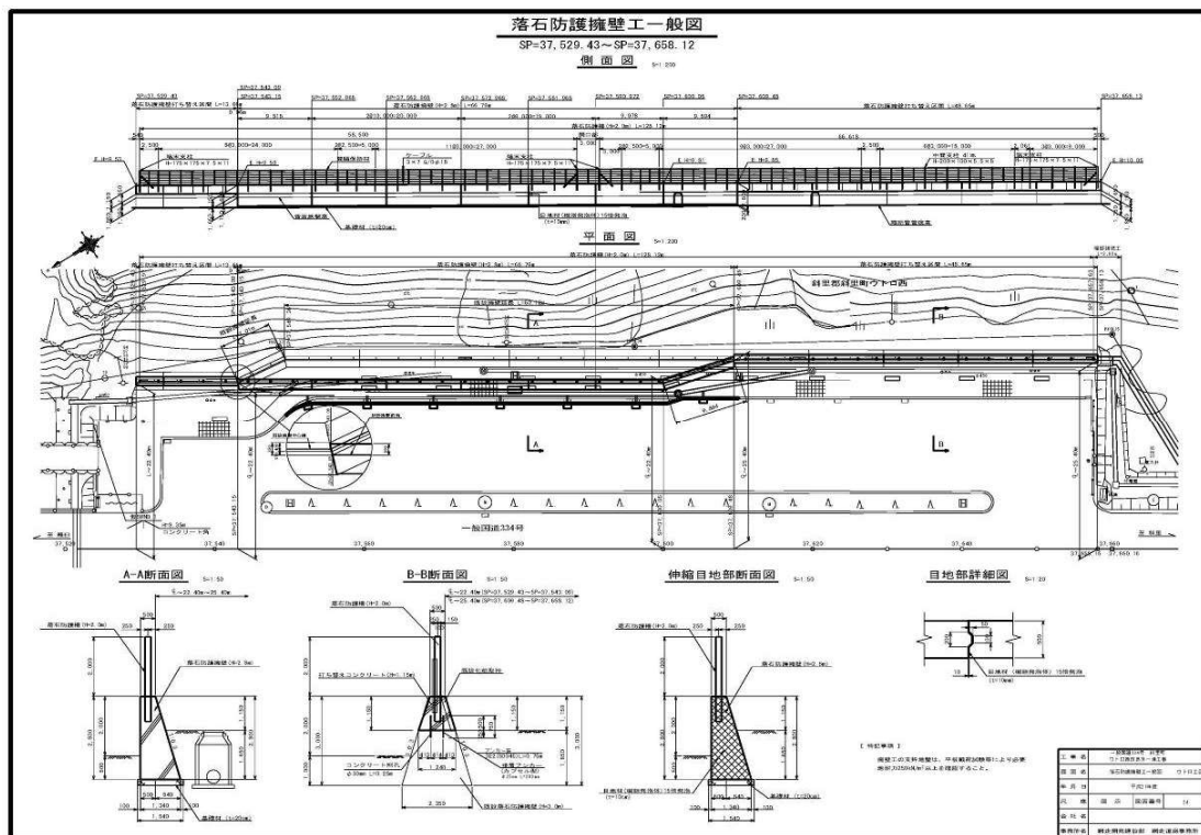
平面図・構造図
