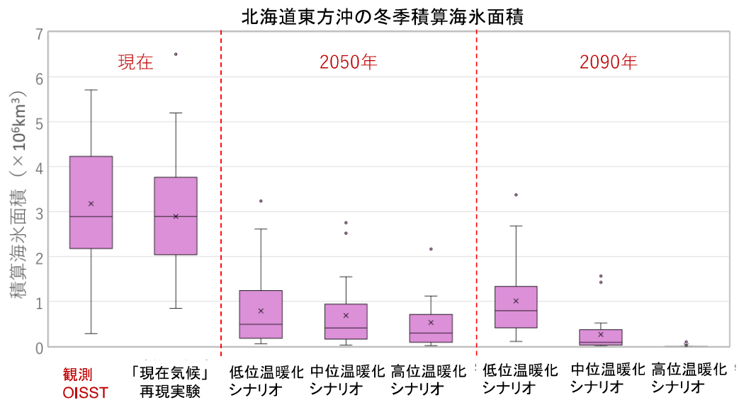
図3 北海道東方海域における冬季積算海氷面積（海氷面積の累計）の「2050年」「2090年」予測の箱ひげ図
