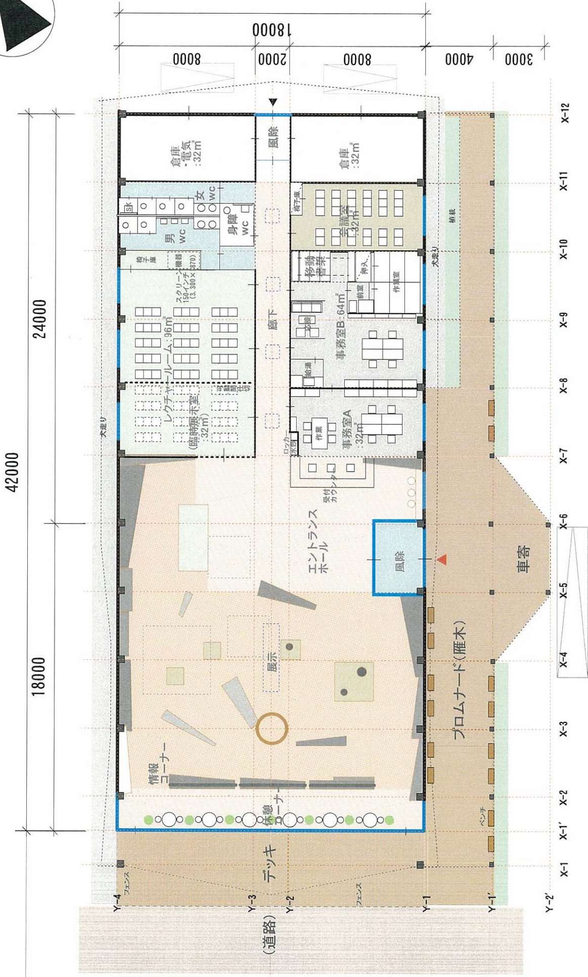
平面図 床面積: 756m 2
