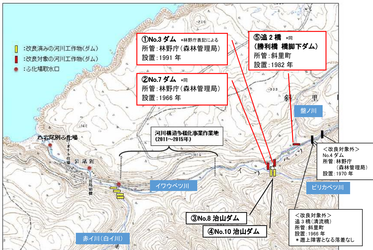
図1: イワウベツ川における改良対象の河川工作物（ダム）位置
