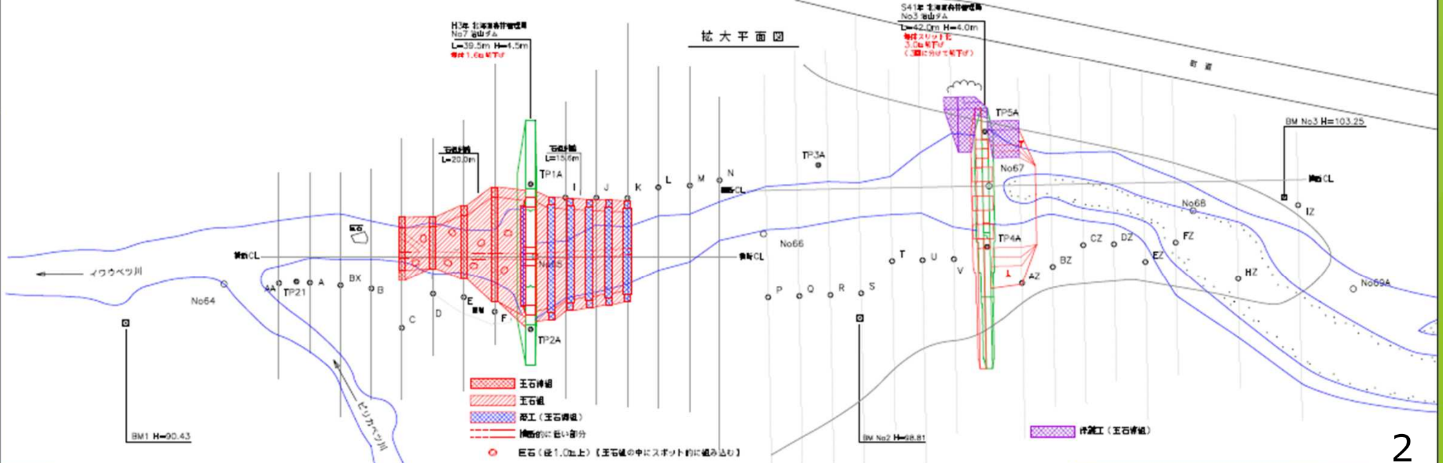
R5改良予定 No 7号ダム
