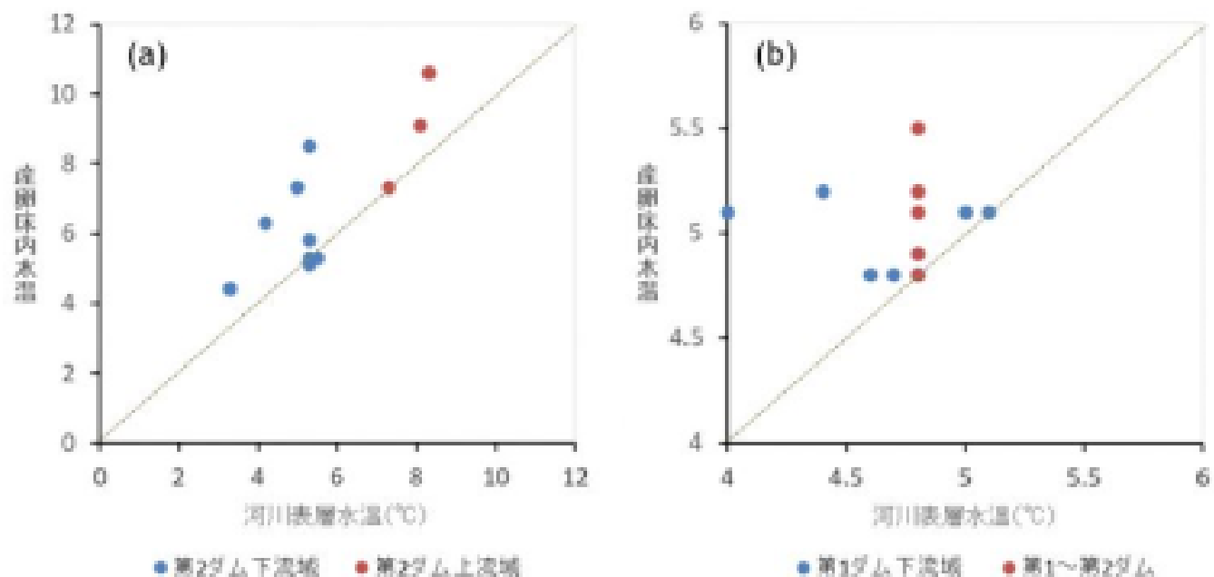
図7 サシルイ川およびチエンベツ川における産卵床内水温と河川表層水温の関係 (a:サシルイ川、b:チエンベツ川)
