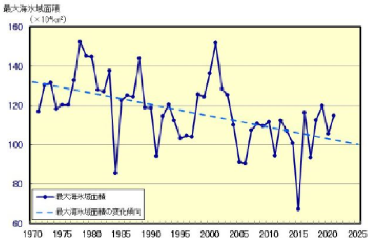
図1 オホーツク海の海水域面積の経年変化(昭和46年～令和3年(1971年～2021年))
